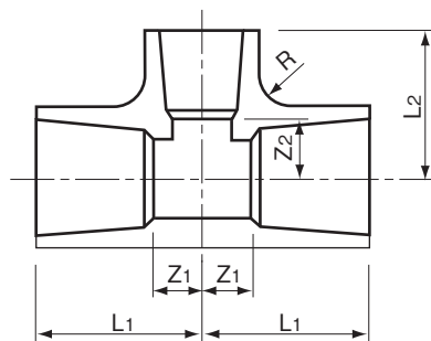
呼び径 13～50mm
